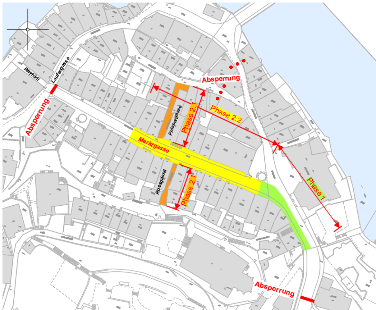
Ausschnitt Bauphasenplan, Stand Januar 2025
